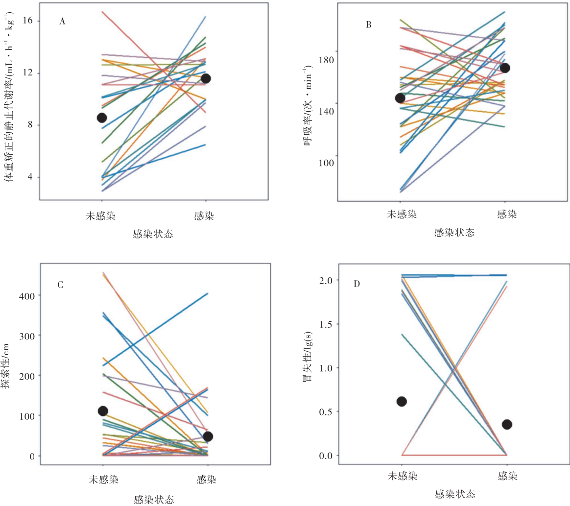
图 2 感染前后高原鼠兔体重矫正的静止代谢率(A)、呼吸率(B)、探索性(C)和冒失性(D)的变化
